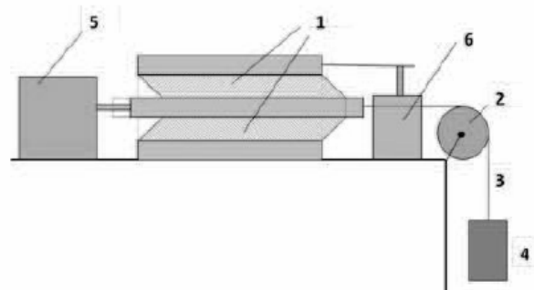
Рис. 1. Схема экспериментальной установки. 1 – слой желатина, 2 – блок, 3 – металлический трос, 4 – ёмкость с водой, 5 и 6 – микрометры.
