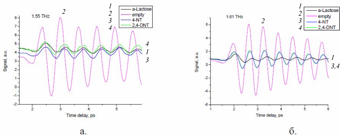
Рис.1. Временные зависимости поля квазимонохроматического терагерцового излучения, прошедшего через пустую подложку ("empty") и подложки с нанесенными веществами. Частота осцилляций поля - а: 1.55 ТГц, б: 1.61 ТГц.
