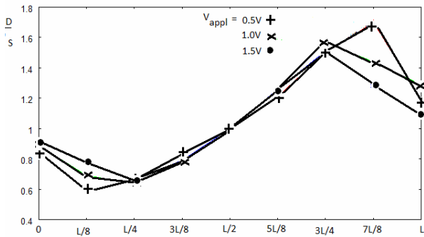
Рис. 2. Зависимость отношения C'D/C'S от расстояния X . L -длина канала. E-mail: timartok@mail.ru
