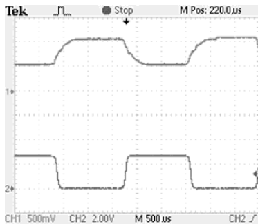
Рис 1. Осциллограмма интенсивности модулированного(сверху) и информационного (снизу) излучений
