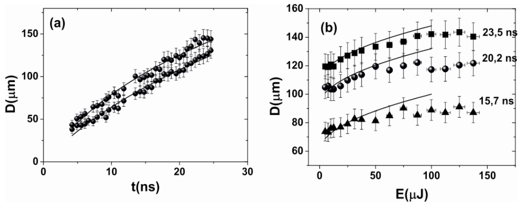
Рис.2. (а) Зависимость диаметра переднего и заднего фронта ударной волны от задержки между возбуждающим и пробным импульсом для энергии лазерного импульса 10мкДж. (b) Зависимость диаметра переднего фронта ударной волны от энергии лазерного импульса для различных времен задержки. Линии показана корневая зависимость.
