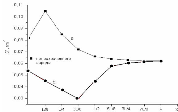
Рис. 1 Зависимость C' от X для случаев встраивания единичного отрицательного (а) и положительного(б) заряда в оксидном слое.
