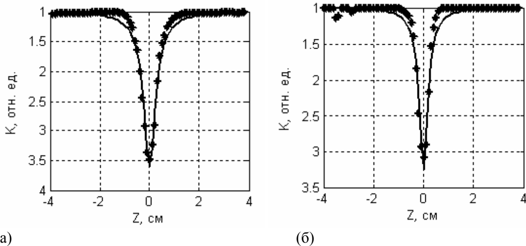
Рис. 1 Кривые Z-сканирования для многослойных углеродных нанотрубок (МУНТ) в диметилформамиде (ДМФА) на длине волны \lambda=532 нм (а), \lambda=1064 нм (б). «*» - экспериментальные данные, «-» - расчетные данные
