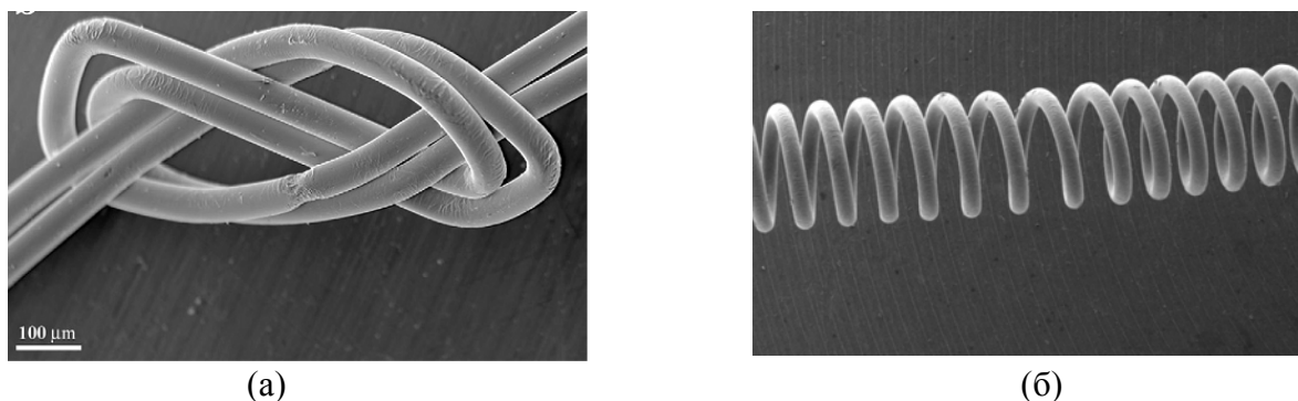
Рис. 1 Изображения толстых Fe_{31}Co_{34}Ni_{10}(SiB)_{25} микропроводов, иллюстрирующих их способностью стягиваться в узел без разрушения (а) и вид пружины диаметром 0.6 мм, демонстрирующая способность микропровода к пластической деформации (б.)
