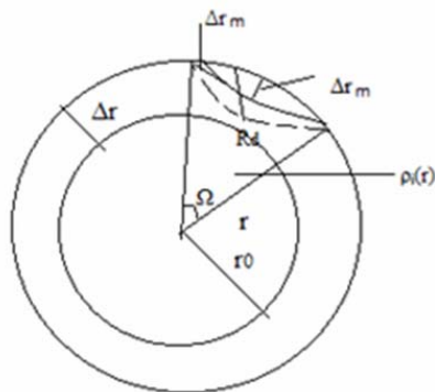
Рис.2. Модель деформированной сферы
