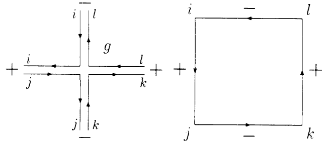
Рис. 2. Соответствие между вершинами и многоугольниками
