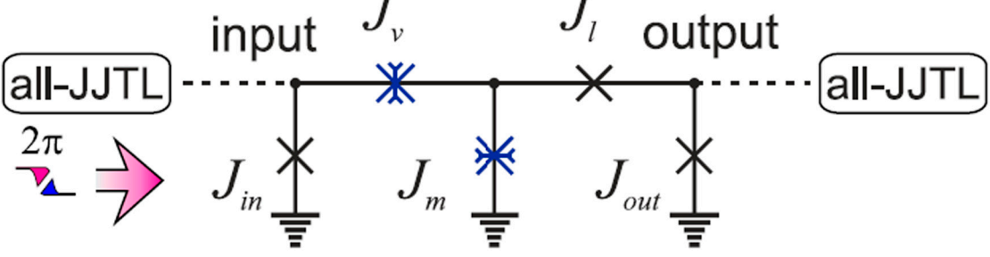
Рис. 2. Пример предложенного безиндуктивного логического блока для сверхпроводниковой цифровой электроники. Крестами на схеме показаны джозефсоновские контакты
