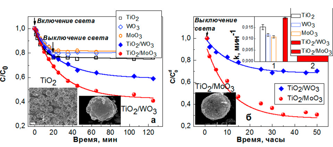
Рис.1 (а) Кинетика разложения на коротких временах родамина 6Ж на поверхности нанокислородов и наногетероструктур в составе микросфер. С 0 соответствует концентрации красителя в момент времени t=0 (свет включен). (б) Дозавременная кинетика деградации родамина 6Ж на поверхности наногетероструктур TiO 2 /V 2 O 5 и TiO 2 /MoO 3 в течение 30 мин при постоянной освещенности в видимом диапазоне. С 0 соответствует концентрации красителя в момент выключения света. Также показаны микрофотографии микросфер из нанокислорода титана, титана/молибдена, титана/вольфрама. На вставке приведены скорости каталитиза для исследуемых образцов
