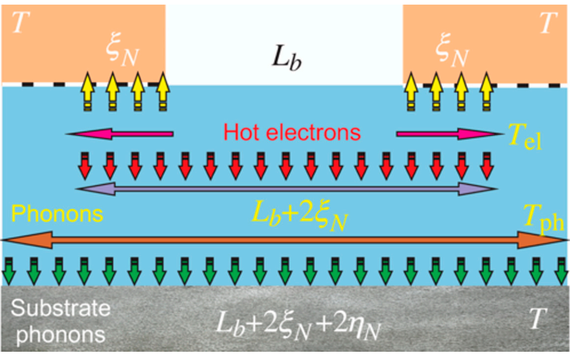
Рис. 1. Пролонгированный джозефсоновский контакт «сверхпроводник — металл — сверхпроводник» в геометрии «мостик переменной толщины», позволяющий получить высокие значения критического тока и сопротивления в нормальном состоянии при высокой воспроизводимости основных характеристик
