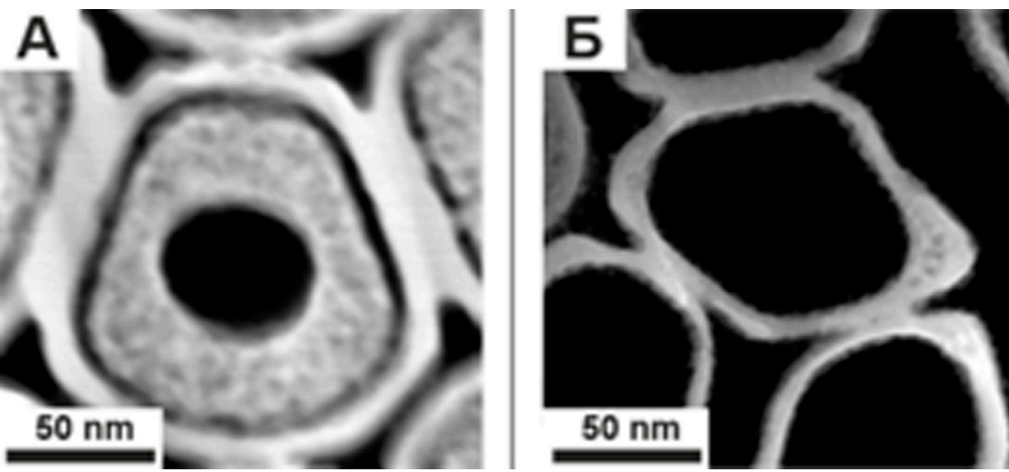
Рис.4 Изображения поверхности многостенных (А) и одностенных (Б) массивов нанотрубок оксида титана, полученные с помощью сканирующей зондовой микроскопии (справ), и микрофотография бокового сканирующего туннельного микроскопа (слева), полученная с помощью сканирующей электронной микроскопии
