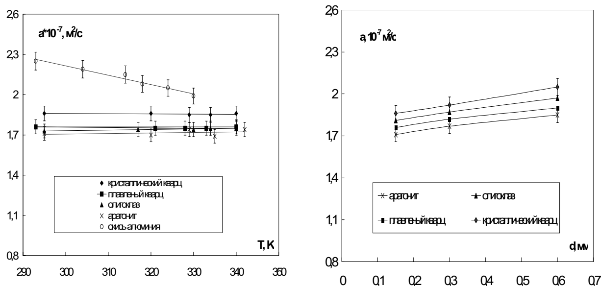
Рис. 1. Поведение температуропроводности исследованных свободных засыпок (а — a_{эфф}(T) для d_1 ; б — a_{эфф}(d) )
