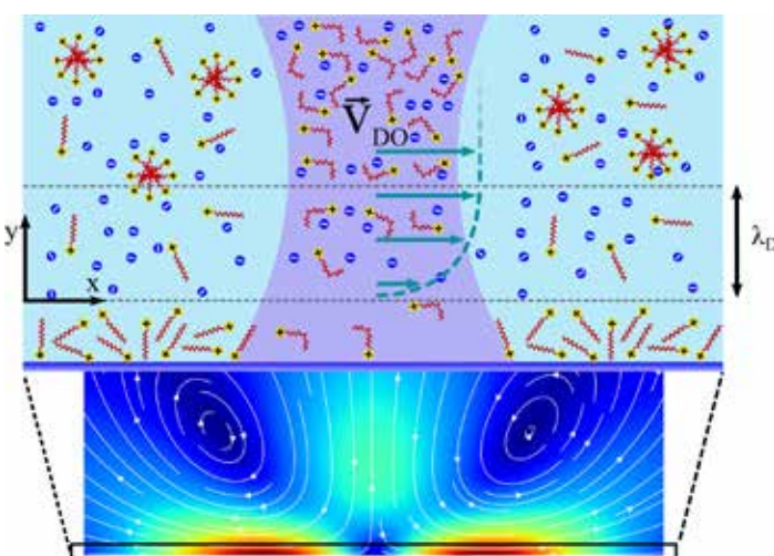
Схема возникновения диффузио-осмотического течения воды из-за перепада концентраций фоточувствительного поверхностно-активного вещества.
