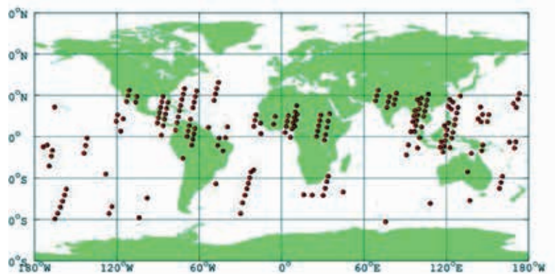
Рис. 9. Карта событий транзитного УФ-свечения в атмосфере Земли по данным первых трех месяцев работы телескопа ТУС.
