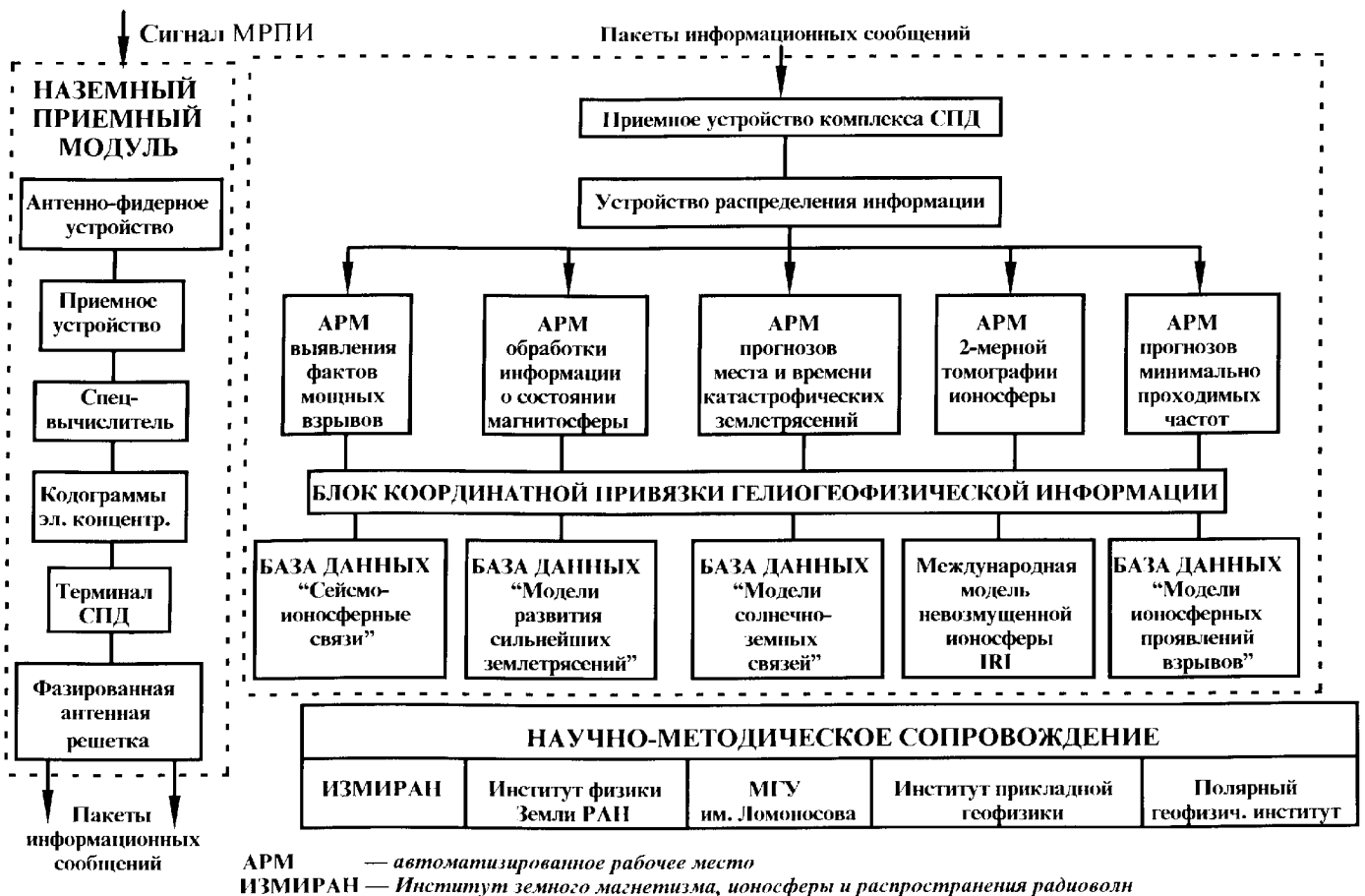
Рис. 2. Наземный пункт обработки информации
