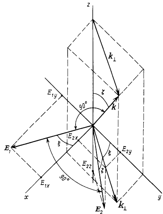
Рис. 2. К вычислению проекций векторов \mathbf{E}_1 и \mathbf{E}_2 , перпендикулярных волновому вектору \mathbf{k} : \mathbf{k}_{\perp} — проекция \mathbf{k} на плоскость xOy . В промежуточных вычислениях можно использовать соотношения \sin \xi = k_x/k_{\perp} , \cos \xi = k_y/k_{\perp} , \sin \zeta = k_{\perp}/k , \cos \zeta = k_z/k
