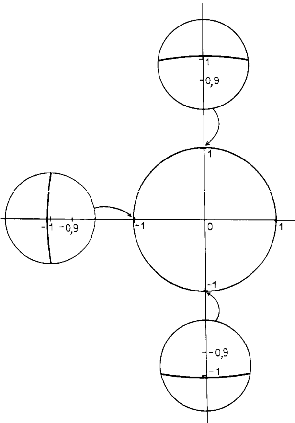
Рис. 1. Траектория электрона от 6-го до 10-го оборота (начальная траектория — круг единичного радиуса)
